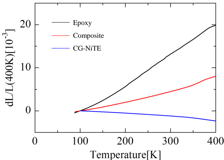
線膨張特性
